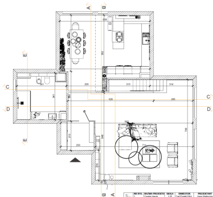
Rys. nr. 1 - RZUT POZIOMY - przekroje proste i przekroje łamane
